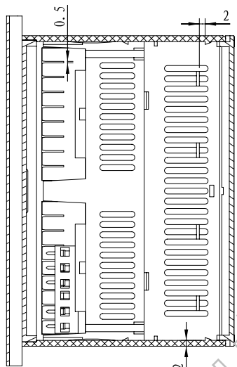
剖面 A-A
