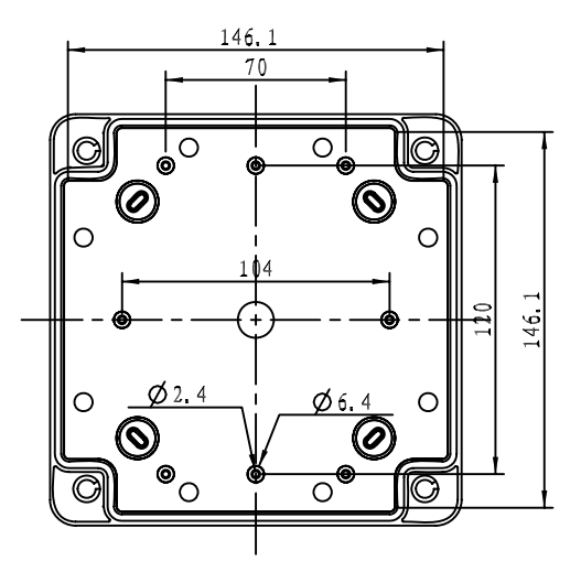
下盖正视图
