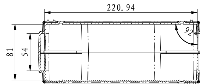
截面 B-B
