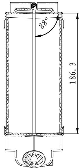
剖面A-A
