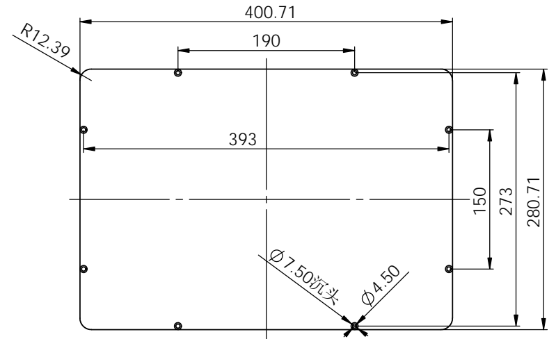
面板尺寸
