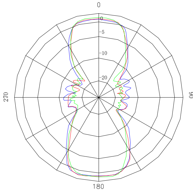
垂直面方向图 Vertical Pattern
