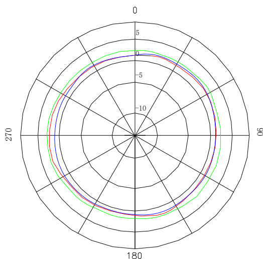
水平面方向图(2.4G天线) Horizontal Pattern
