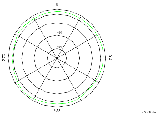
水平面方向图 Horizontal Pattern
