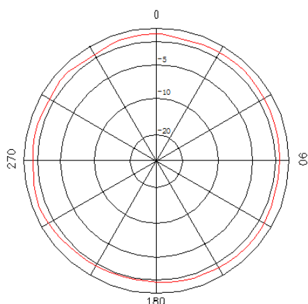
水平面方向图 Horizontal Pattern
