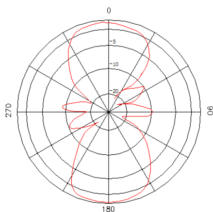
垂直面方向图 Vertical Pattern
