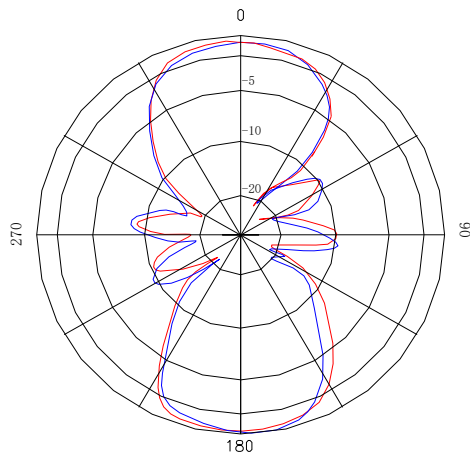
垂直面方向图 Vertical Pattern
