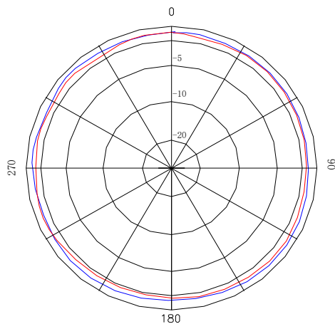
水平面方向图 Horizontal Pattern
