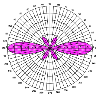
垂直方向图
