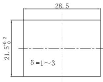
安装面板尺寸 PANEL CUT-OUT
