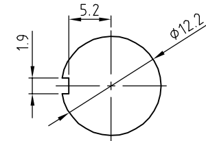
安装面板尺寸 PANEL CUT-OUT
