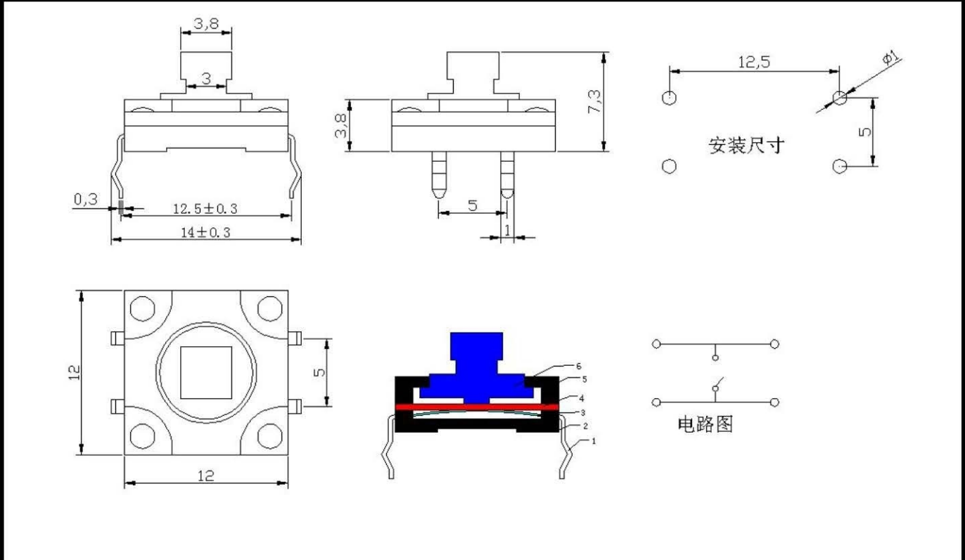
尺寸外型图
