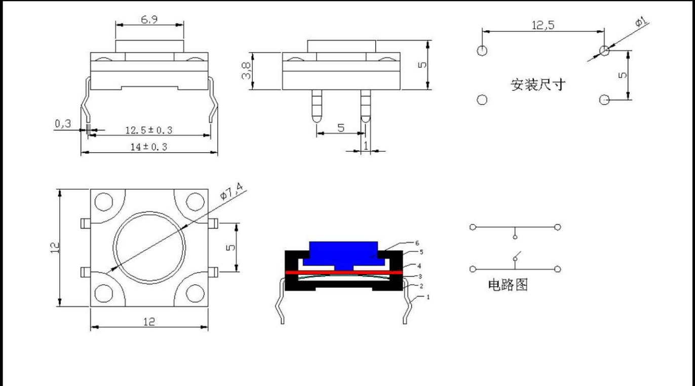
尺寸外型图
